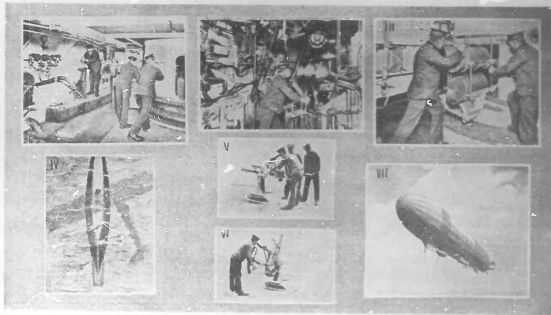
La Guerra Europea. Alimentación de los grandes cañones de un acorazado. I.—Cámara de introducción de proyectiles en la cámara. II.—Mecanismo de alimentación de dos cañones de 12 pulgadas en la cámara directora de un "dreadnought", que sigue el movimiento de ambas piezas. III.—Cerro elevador de cordita, con cartuchos de media carga para un cañón de 12 pulgadas. IV.—Las naves submarinas contra las naves aéreas. Aspecto del submarino sumergido, descubierta por el observador aéreo. V.—El cañón del submarino apuntando contra una nave aérea. VI.—El cañón apuntando en la línea normal de tiro. VII.—El dirigible alemán Schwaben, tipo Zeppelin.
